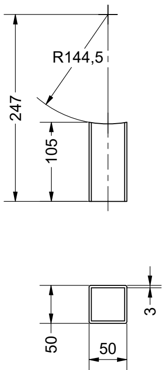
Pos. 2 ( 1 : 5 )
