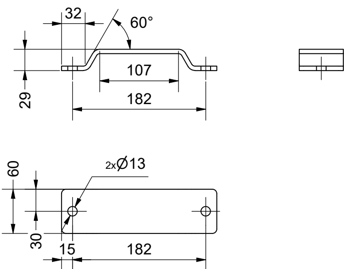
Pos. 1 ( 1 : 5 )
