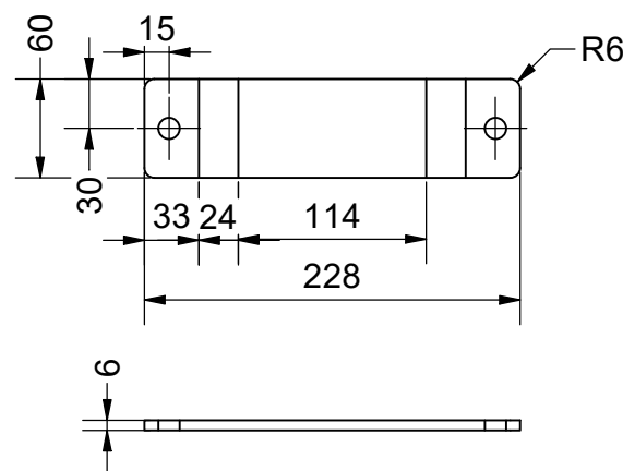
Pos. 1 Flat pattern ( 1 : 5 )
